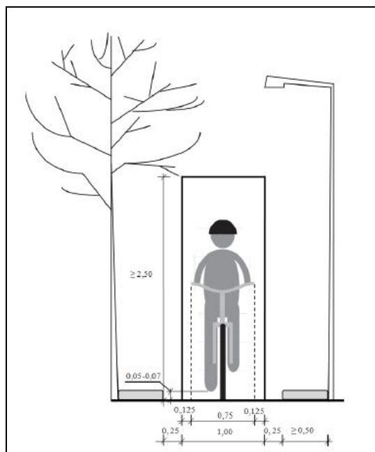
5 pav. Pagrindiniai dviratininkų eismui reikalingi gabaritai
