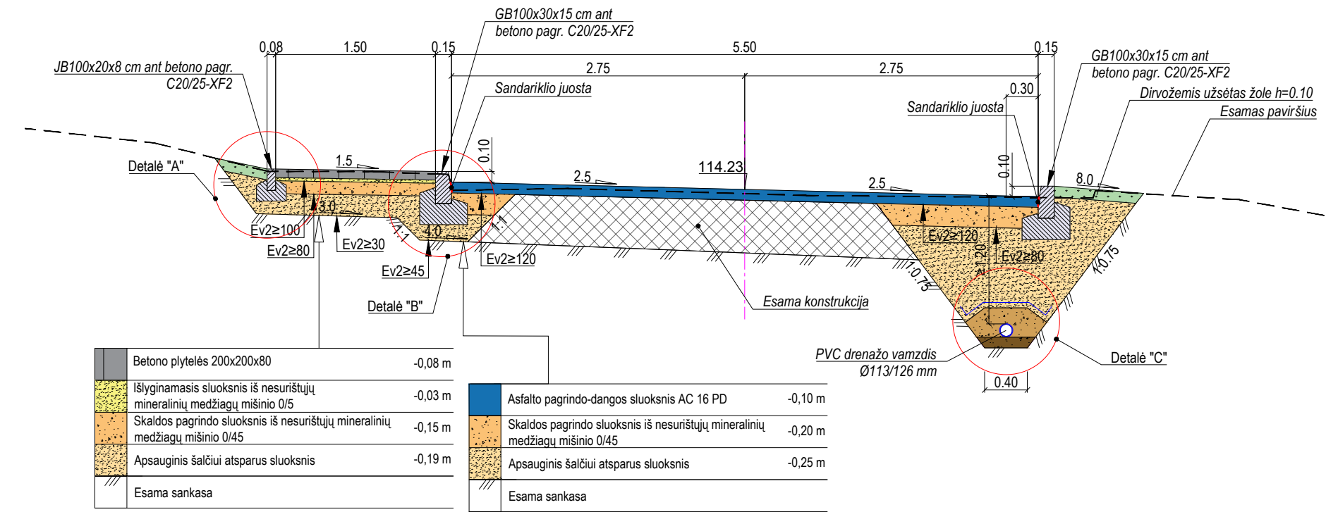
SKERSINIS PJŪVIS M 1:50 Pk. 0+40
