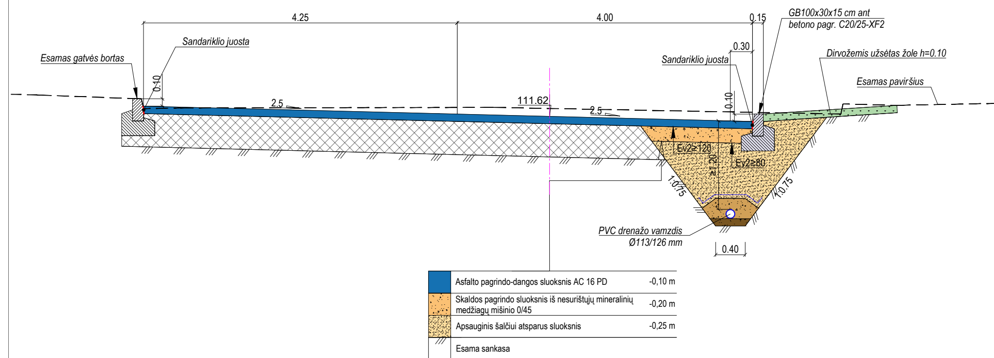
SKERSINIS PJŪVIS M 1:50 Pk. 1+60
