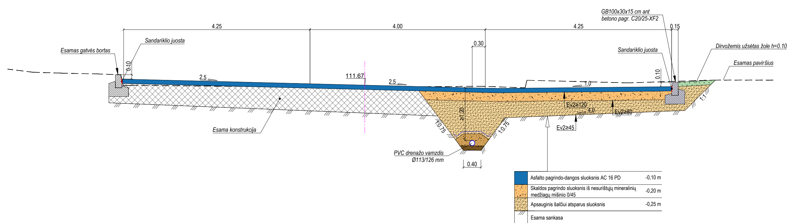
SKERSINIS PJŪVIS M 1:50 Pk. 1+85
