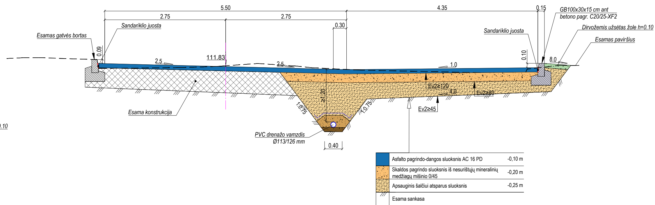
SKERSINIS PJŪVIS M 1:50 Pk. 1+15
