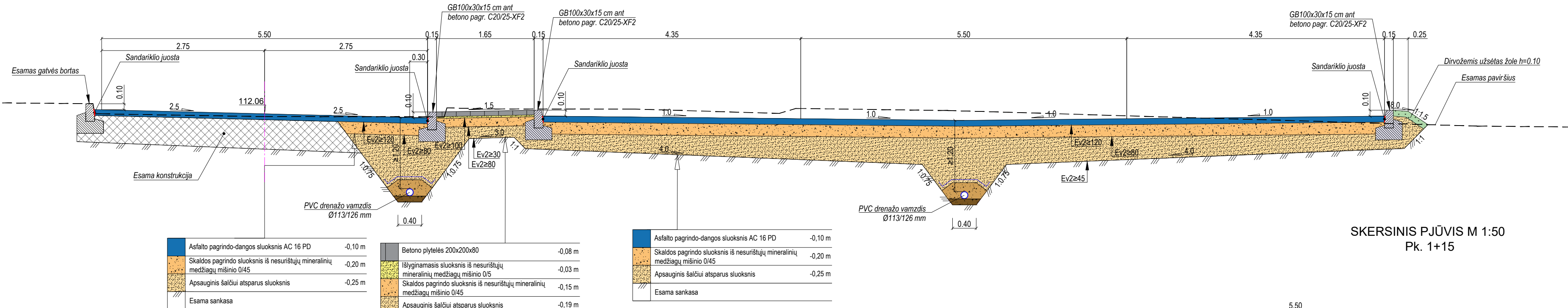
SKERSINIS PJŪVIS M 1:50 Pk. 1+00
