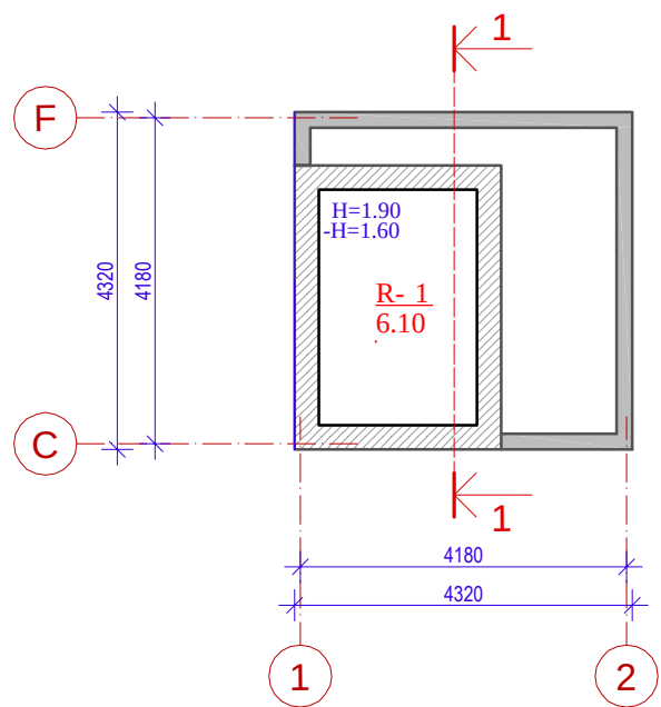
ESAMO RŪŠIO IR ESAMŲ PAMATŲ PLANAS M 1:100
