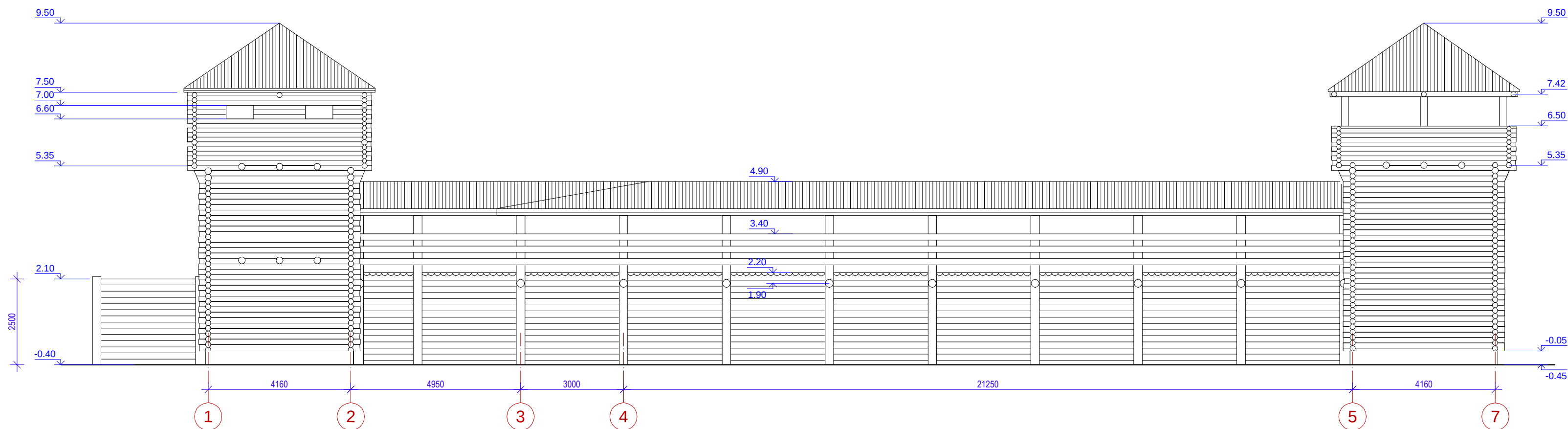
PIETRYTINIS (J. BILIŲ NO GAVĀS) FASADAS M 1:100
