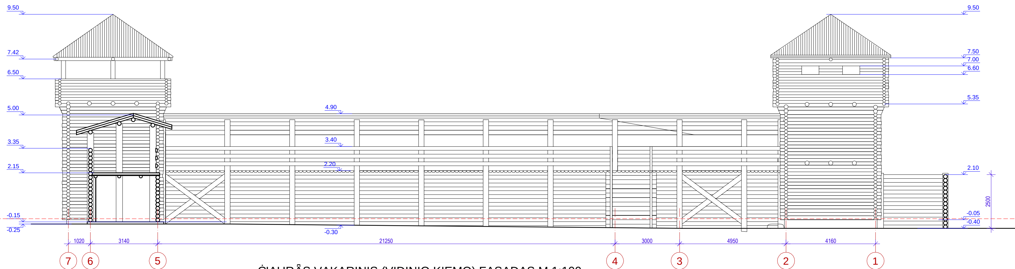
ĢIAURĀS VAKARINIS (VIDINIO KIEMO) FASADAS M 1:100
