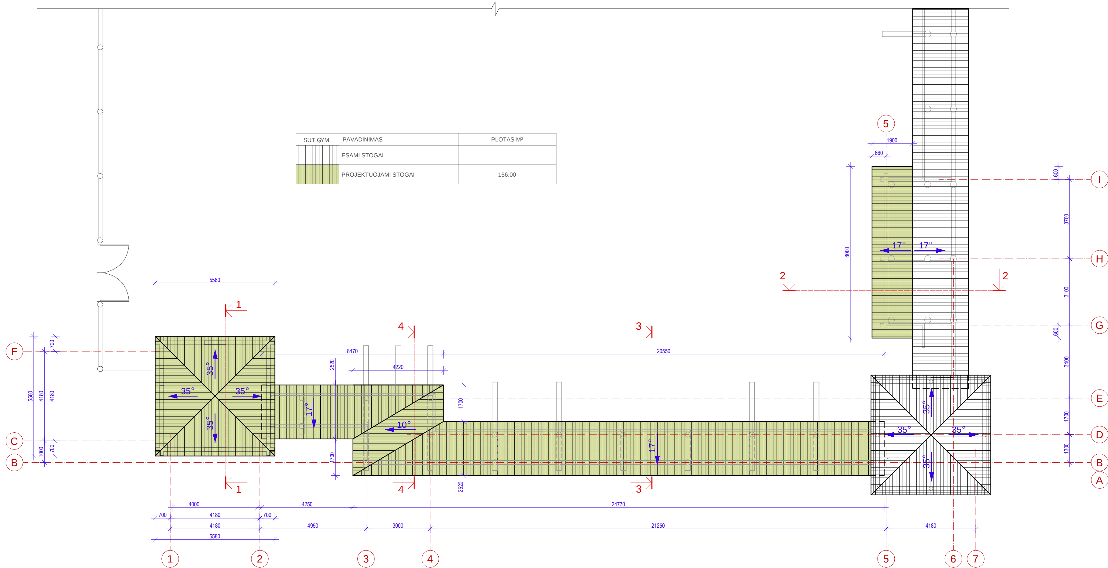
STOGO PLANAS M 1:100
