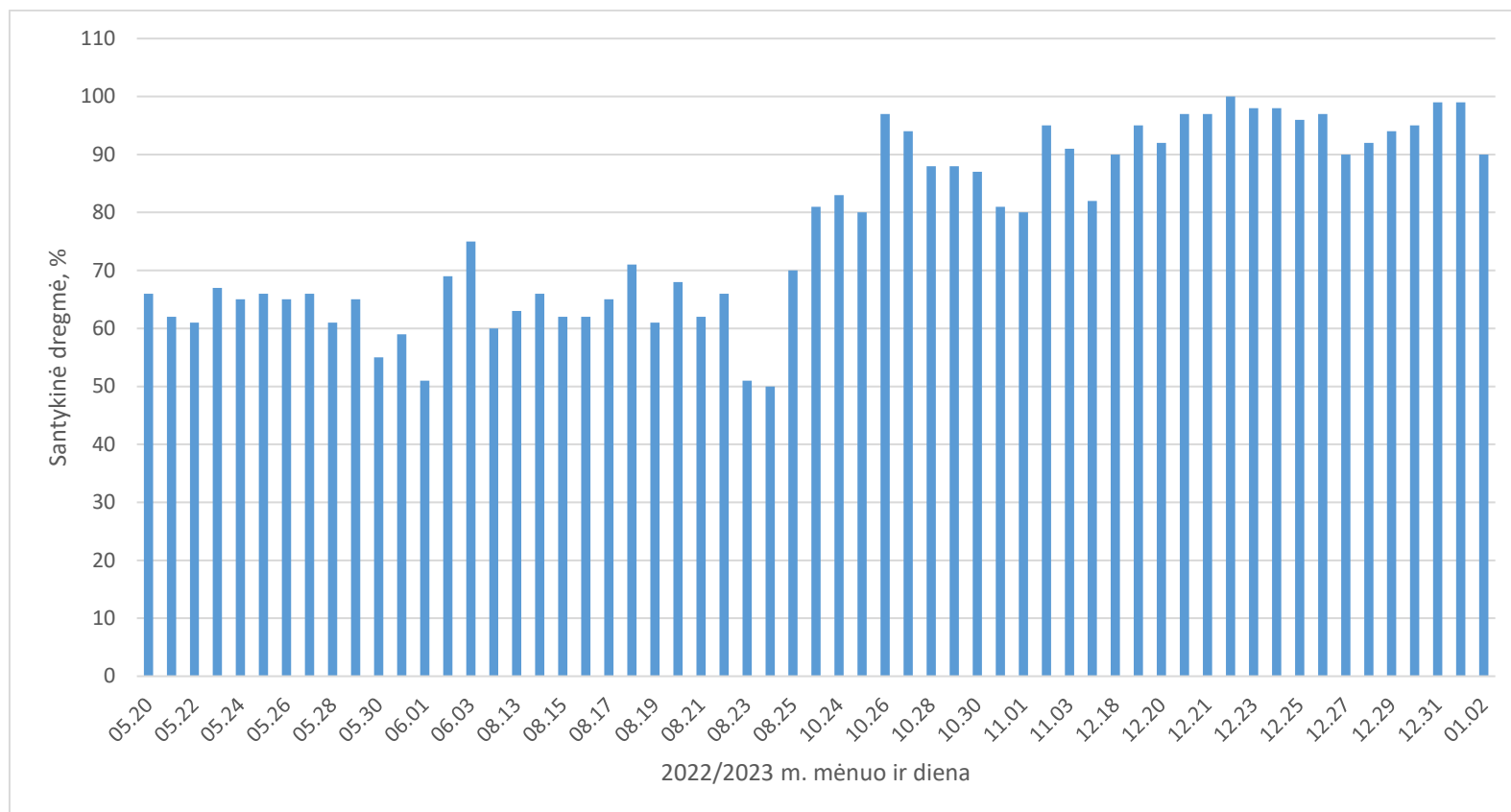
Grafikas Nr. 3 Santykinė drėgmė
