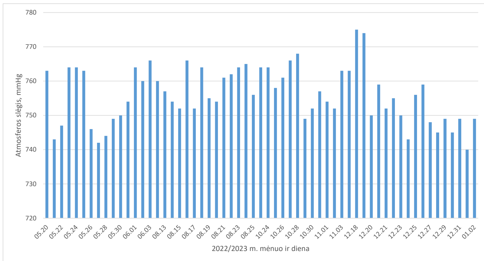
Grafikas Nr. 2 Atmosferos slėgis
