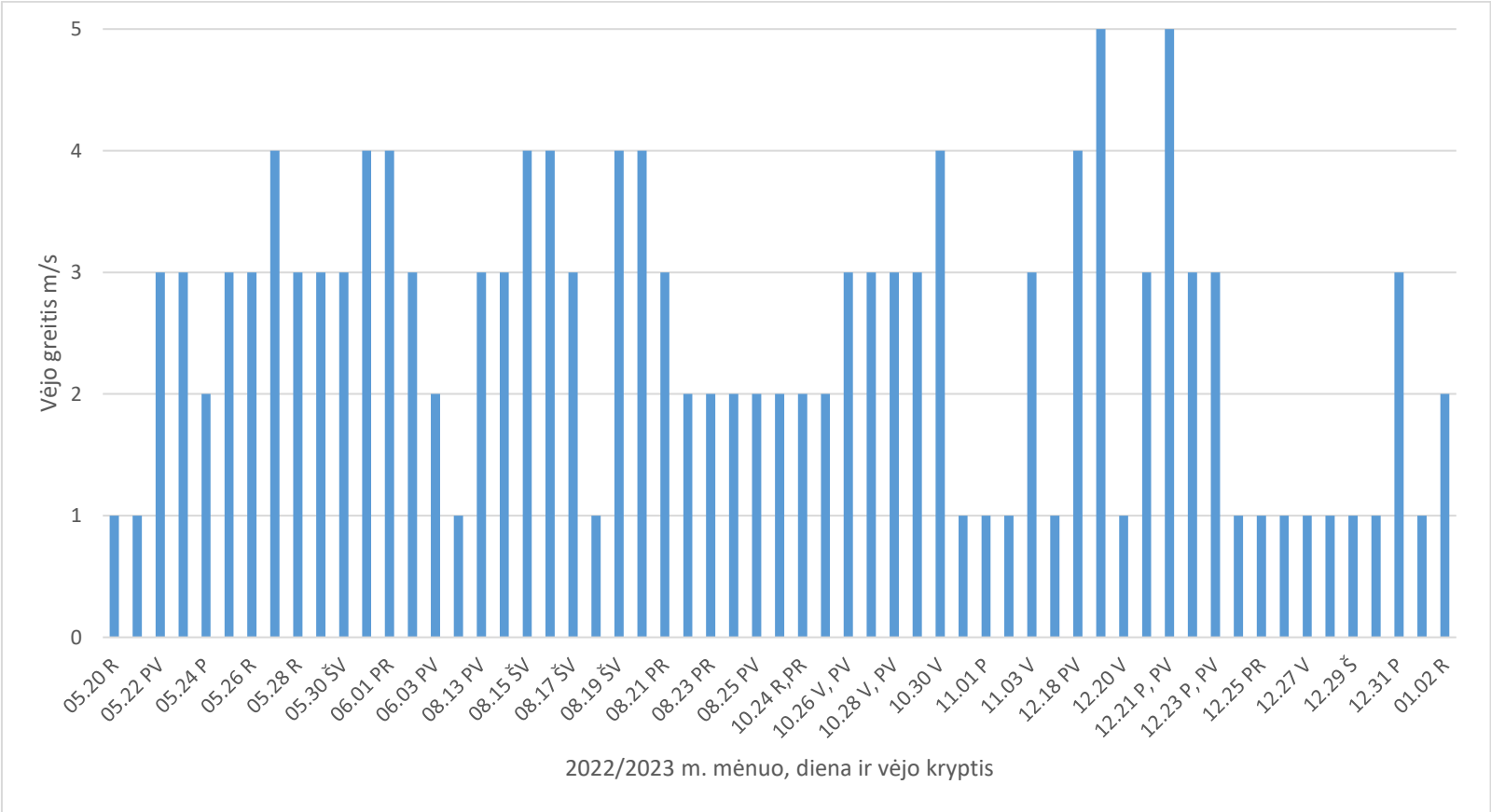
Grafikas Nr. 1 Vėjai ir jų kryptis
