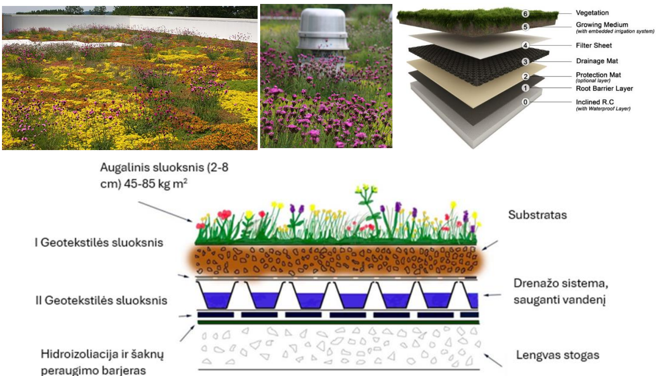
25 pav. Preliminarus stogo sluoksnių planas, kuris tikslinamas detaliojo planavimo metu. Šaltiniai.
