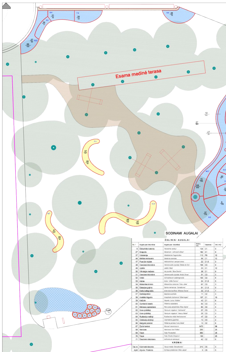
43 F pav. Lokacija Nr. 6 A.Baranauskos aikštė.. Žalinimo sprendinių schema. Šaltinis – sudaryta autorių
