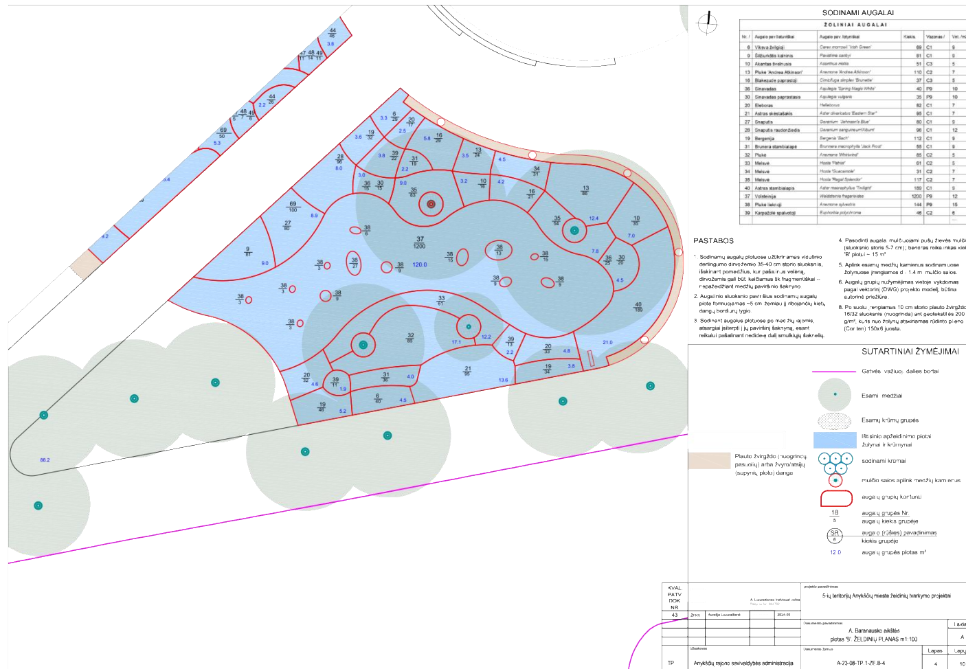
43 E. pav. Lokacija Nr. 6 A.Baranausko aikštė. Žaliniojo sprendinių schema. Šaltinis – sudaryta autorių
