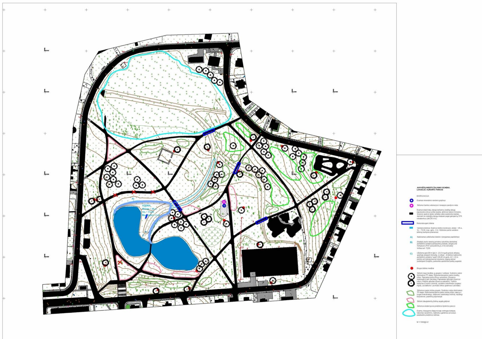
14 pav. Lokacija Nr. 1. Miesto parkas. Žaliniojo sprendinių schema. Šaltinis – sudaryta autorių.
