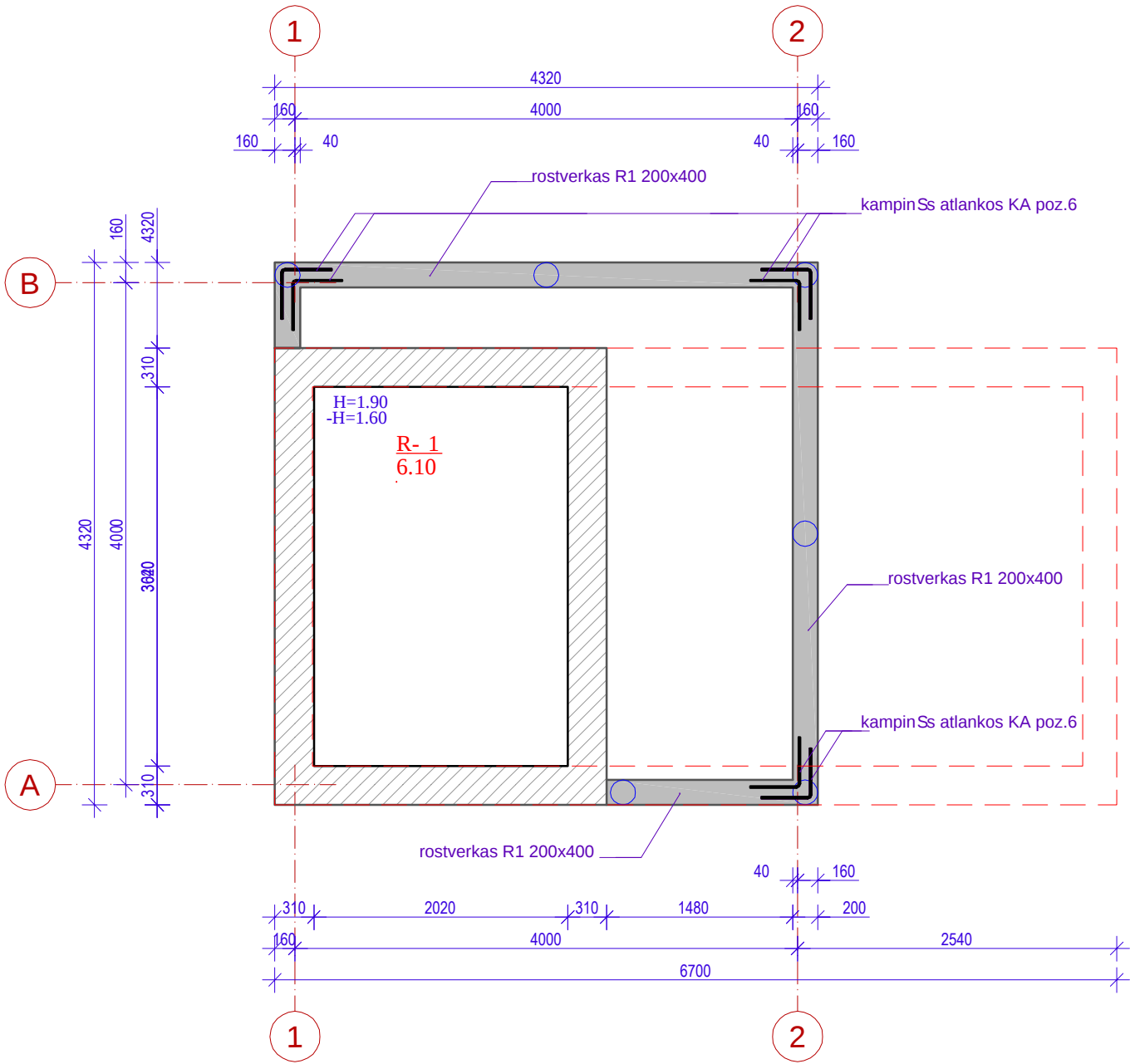
EASAMr PAMATr , ROSTVERKO R1 IR RŲSIO PLANAS M1:50
