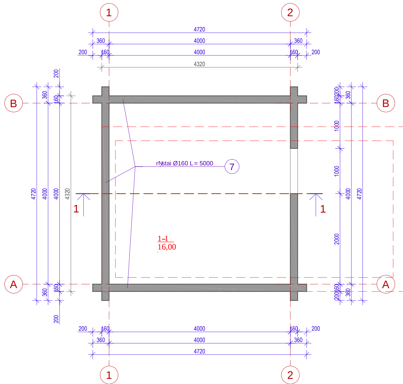
AUKŲTO PLANAS M1:50
