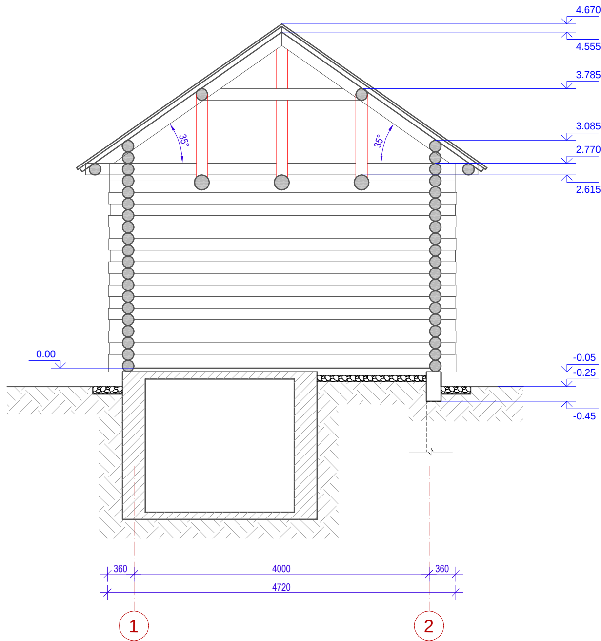
PJŲVIS 1-1 M1:50
