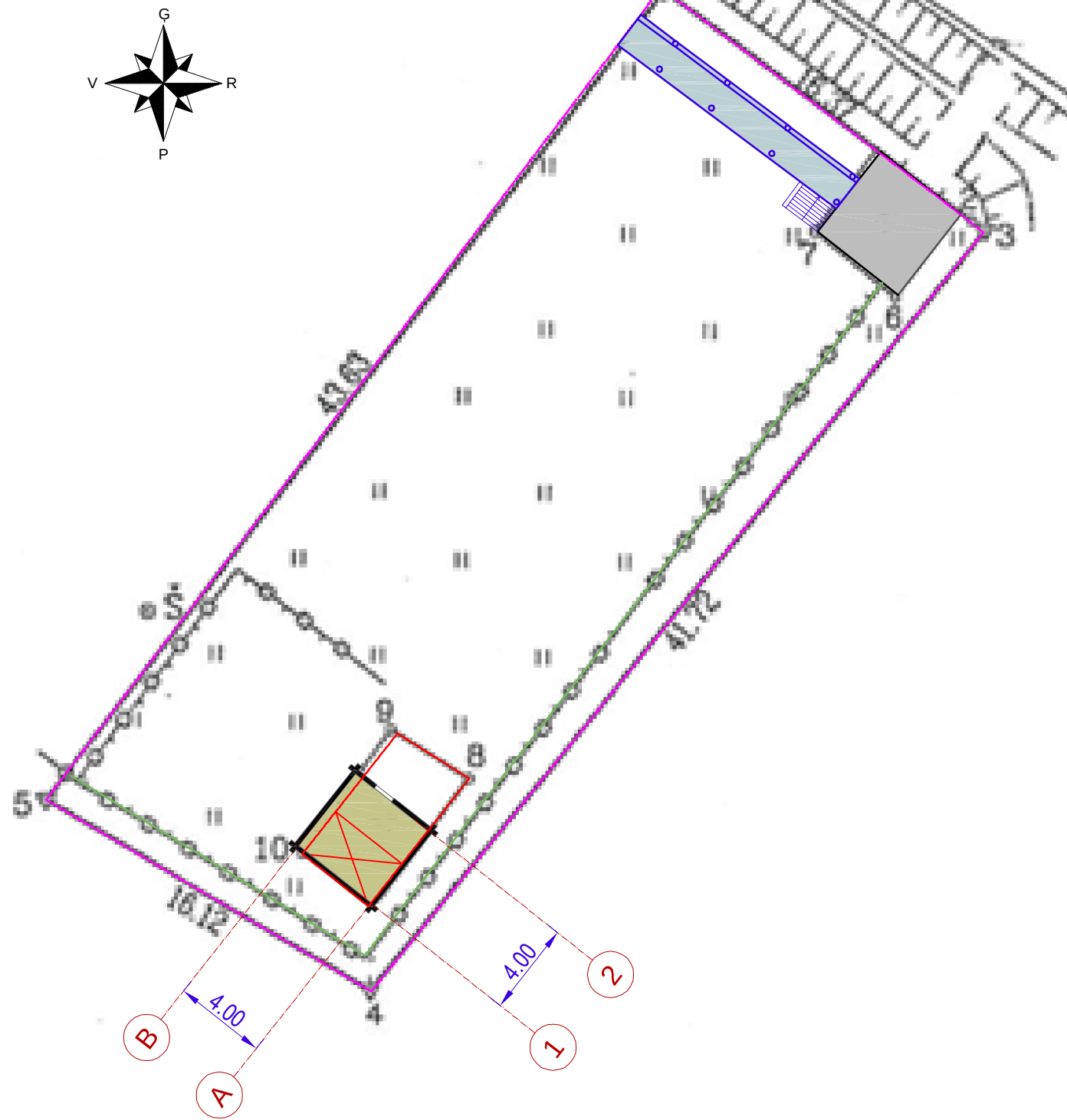
SITUACIJOS PLANAS
