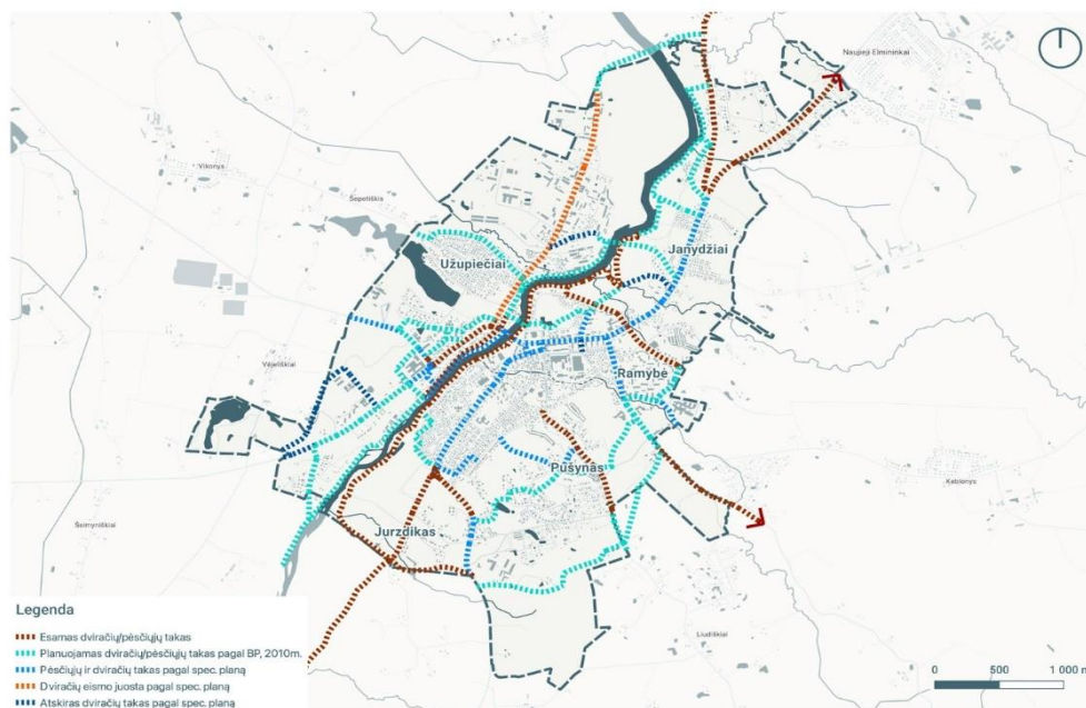
85 paveikslas. Esama ir planuojama dviračių ir pėsčiųjų takų infrastruktūra Anykščių mieste
