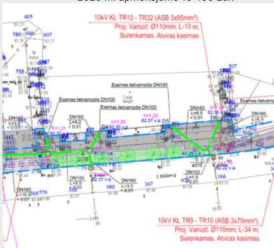
Inžinerinių tinklų plano ištrauka
