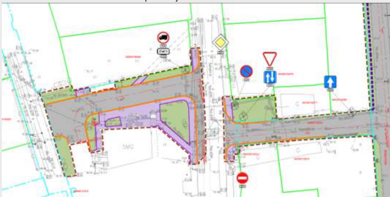
Jvažiavimo nuo Šaltupio g. (akligatvio) sprendiniai pagal žalinimo planą
