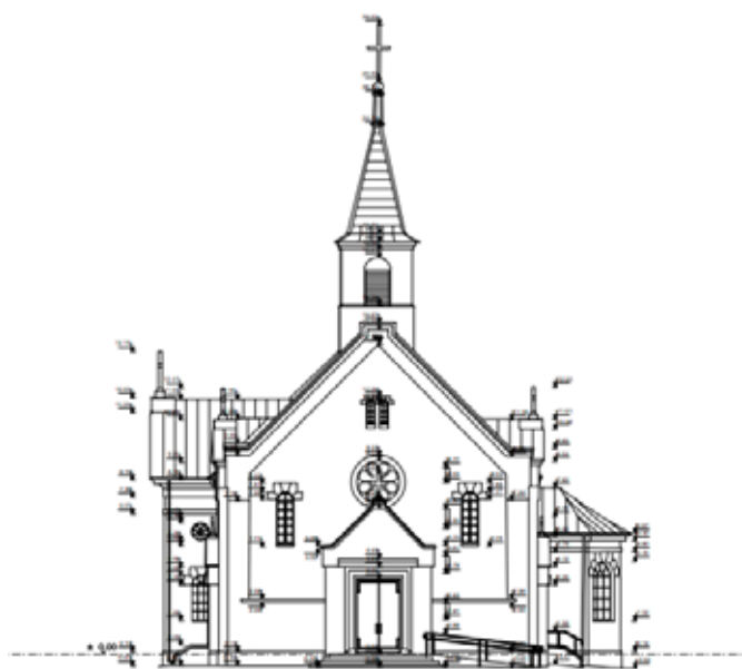
Andrioniškio bažnyčios fotogrametriniai apmatavimai, 2023 m.
