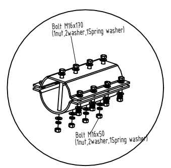
Vamzdžio jungties detalė
