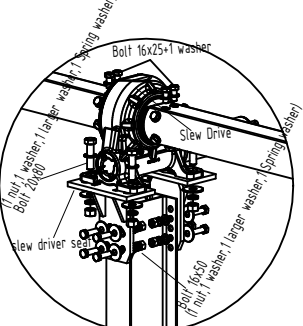
Pavaros montavimo detalė
