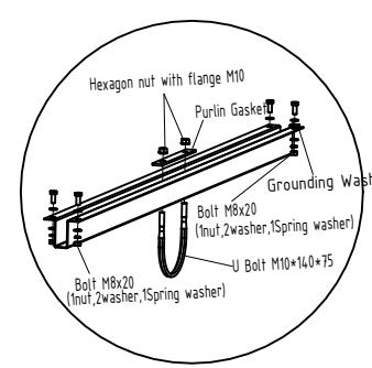
Modulio tvirtinimo detalė
