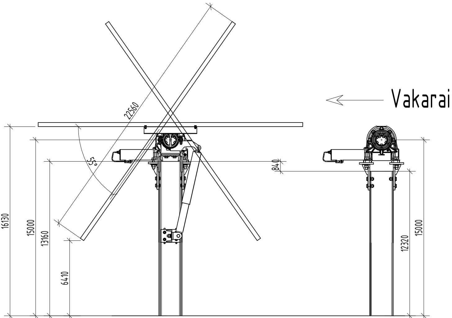
Pjūvis 1-1
