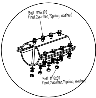
Vamzdžio jungties detalė
