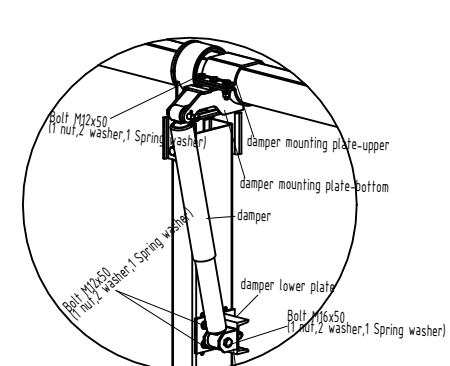
Sklendės tvirtinimo detalė
