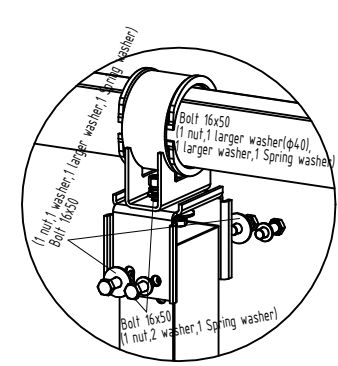
Postamento tvirtinimo detalė
